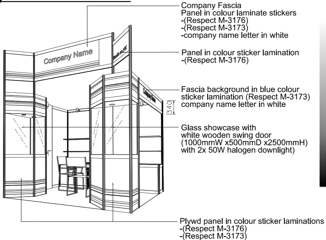
PERSPECTIVE N.T.S.
